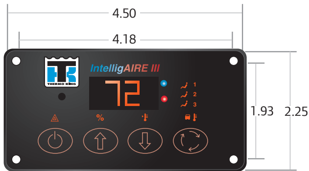
Display Module
